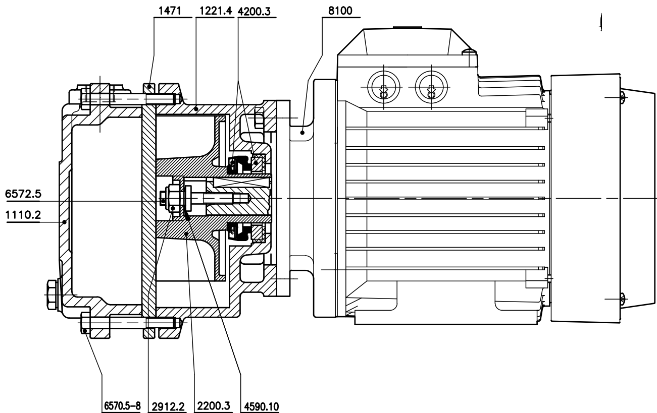
Independet priming pump Bomba de autocebado independiente
